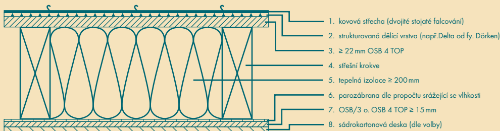
vzduchotěsná střešní konstrukce
